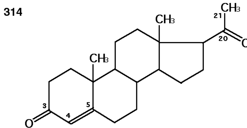
Progestérone
