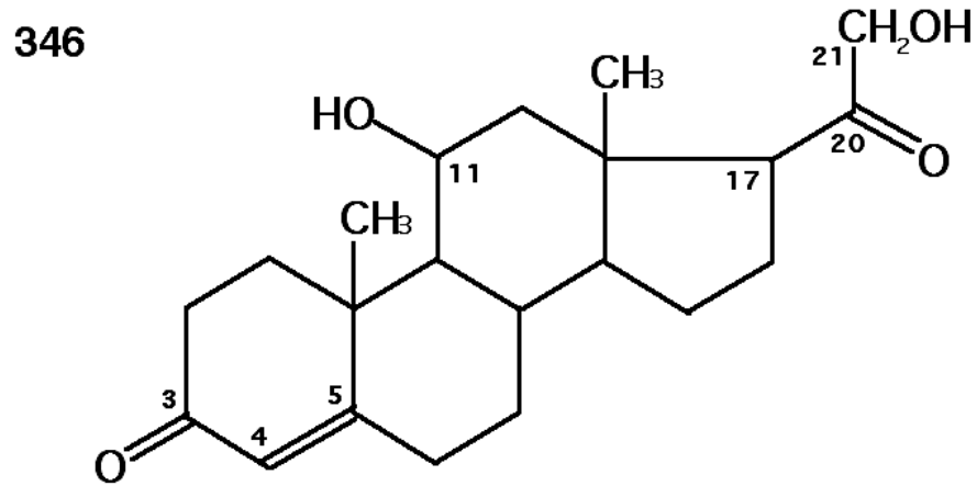
Corticostérone
