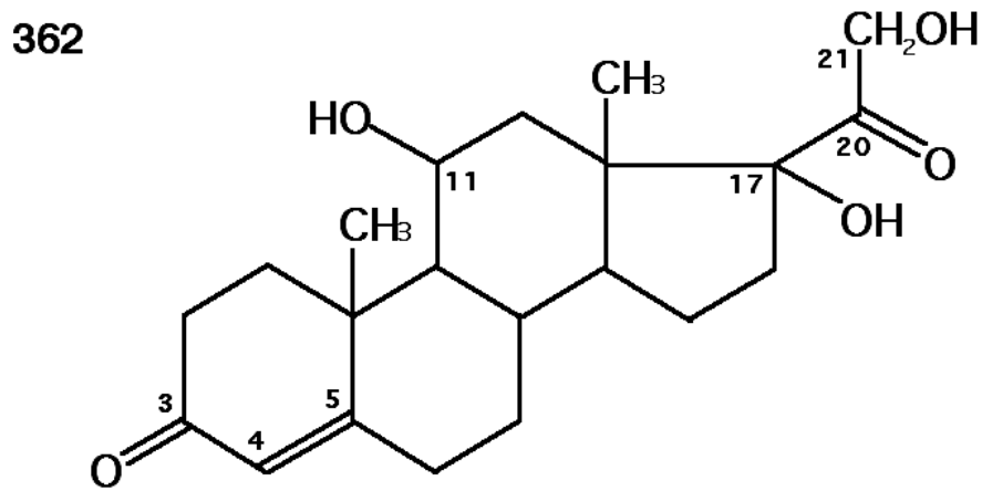
Cortisol
