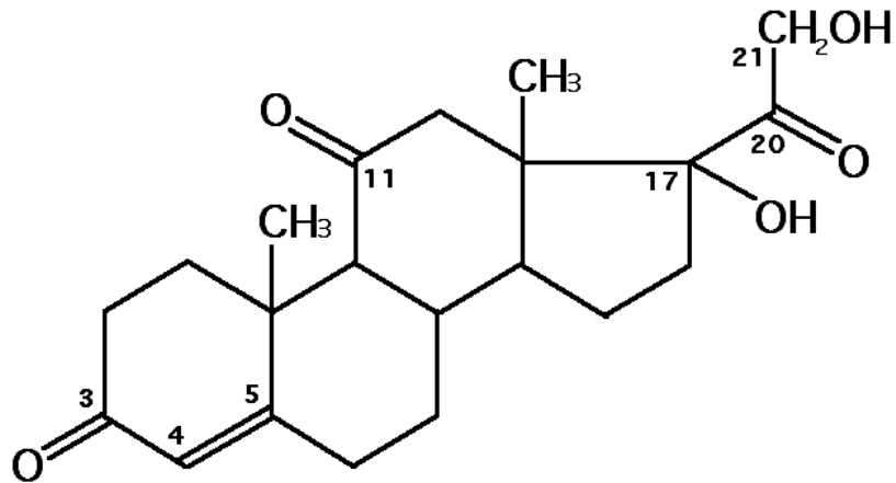
Cortisone
