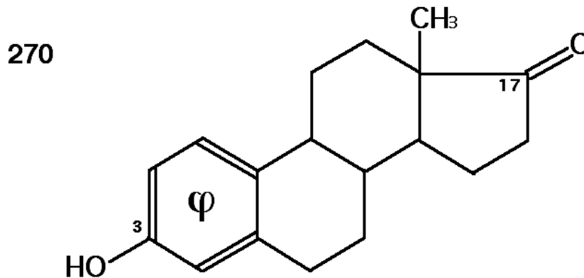
Œstrone
